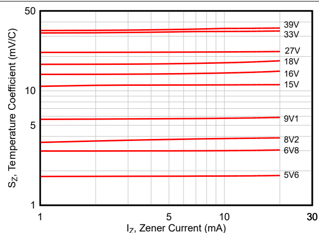
図 6-2. 温度係数
