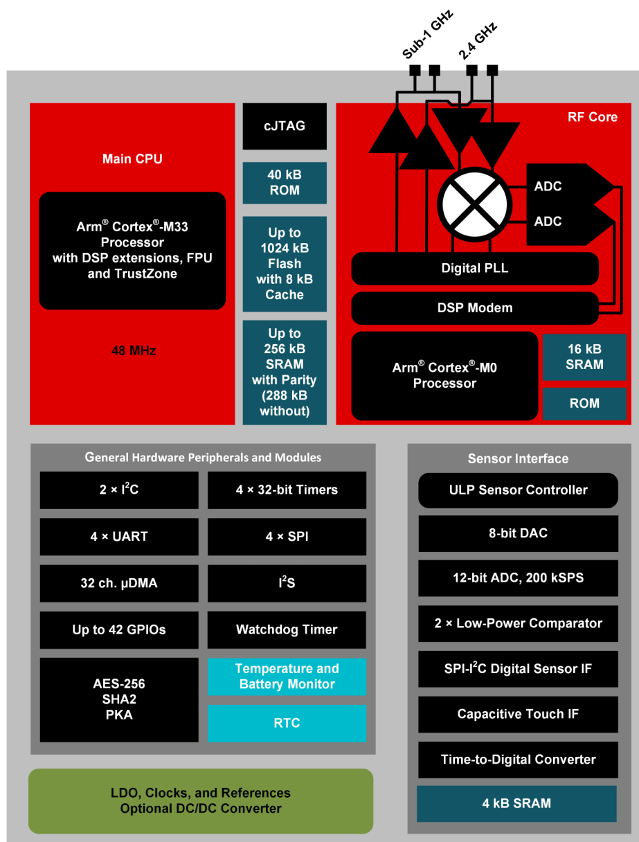
CC1354R10 ブロック図
