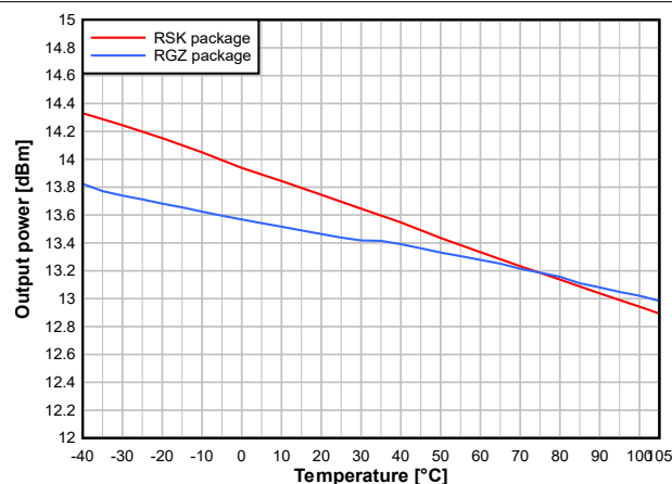
図 7-25. Output Power vs. Temperature (50kbps, 868.3MHz, +14dBm)
