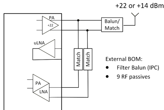
図 8-2. スイッチレス デュアル PA リファレンス デザイン
