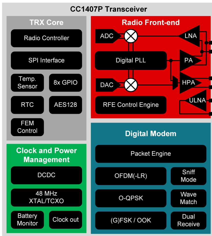
CC1407P ブロック図
