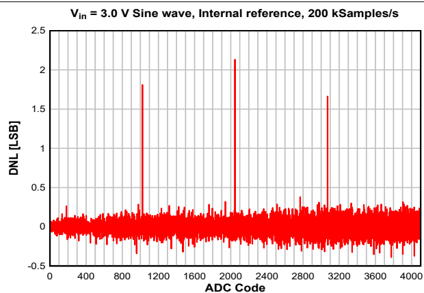
図 7-36. DNL vs. ADC Code
