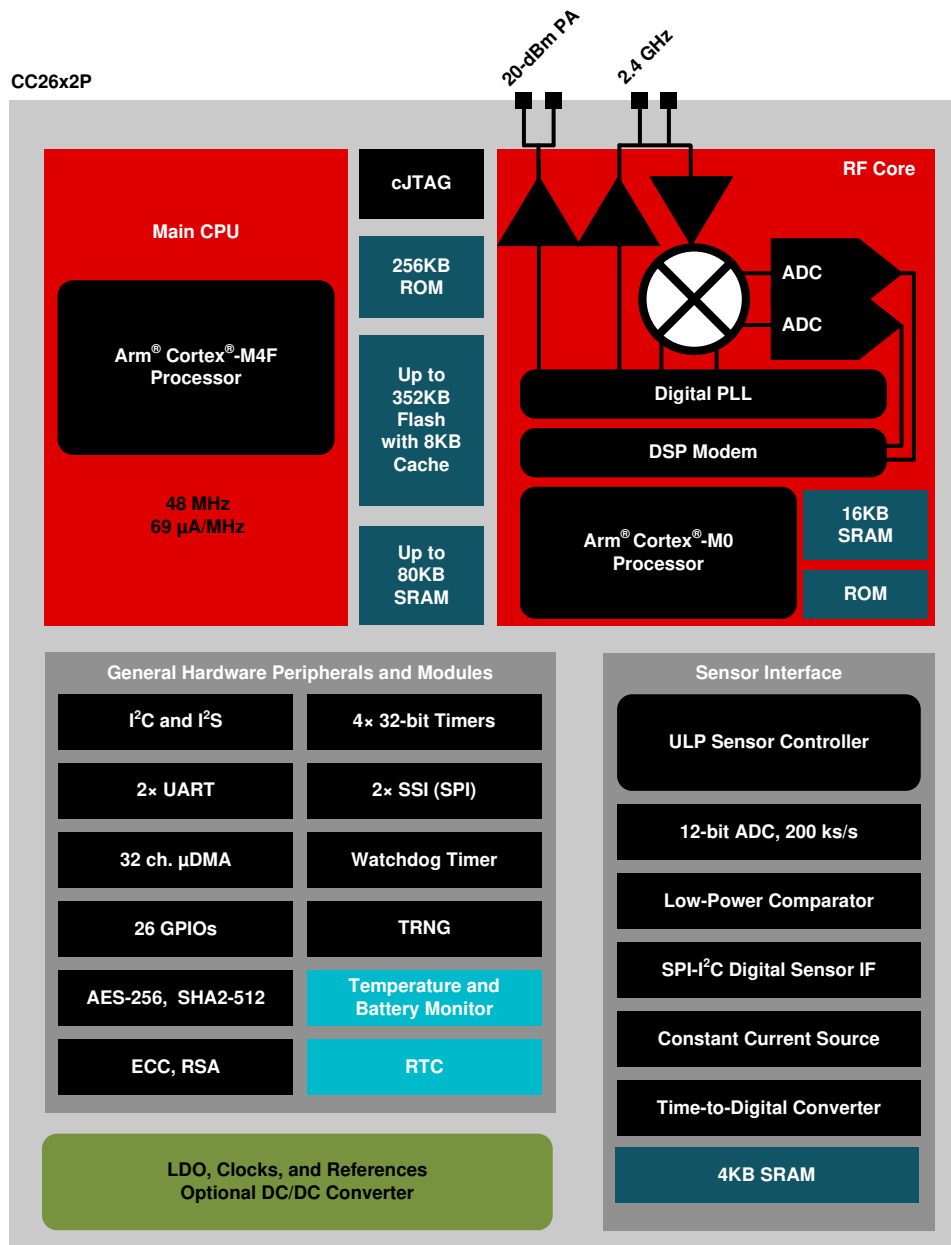
CC2652P ブロック図
