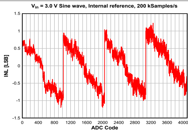
図 7-35. INL vs. ADC Code
