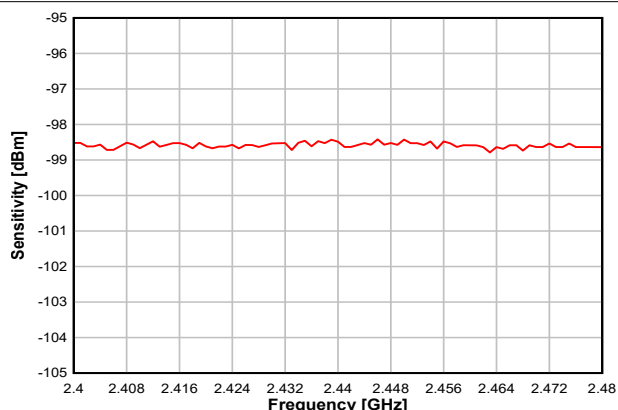
図 8-11. Sensitivity vs. Frequency (IEEE 802.15.4-2006, 250 kbps, OQPSK DSSS 1:8, 2.44 GHz)
