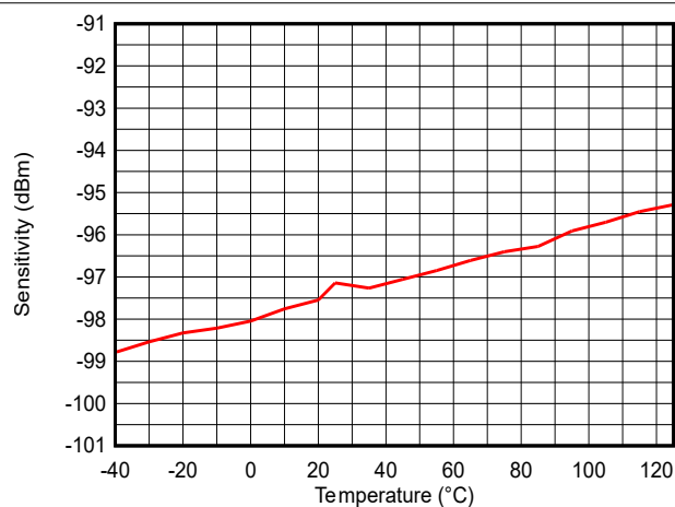
図 7-16. 感度と温度との関係 (LE 1M PHY、2.44GHz)
