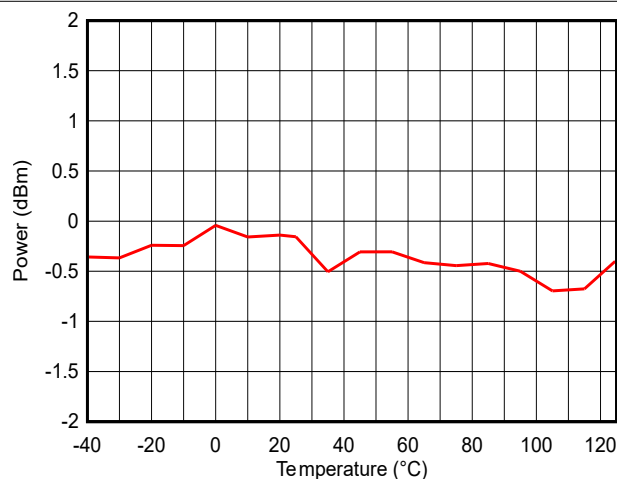
図 7-22. 出力電力と温度との関係 (LE 1M PHY、2.44GHz、0dBm)
