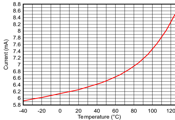
図 7-8. RX 電流と温度との関係 (LE 1M PHY、2.44GHz)、 V_{DD5} = 3.3\text{V}
