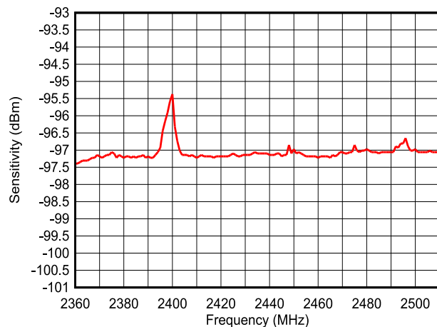
図 7-14. 感度と周波数との関係 (LE 1M PHY)
