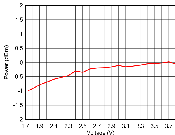
図 7-24. 出力電力と電源電圧 (VDDS) との関係 (LE 1M PHY、2.44GHz、0dBm)
