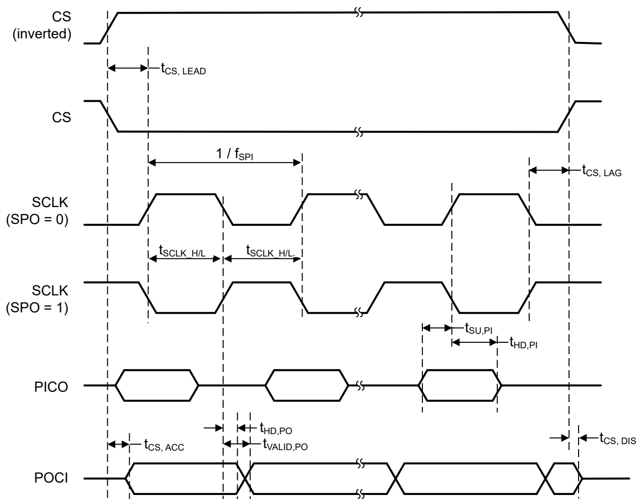
図 7-3. SPI のタイミング図 — ペリフェラル モード、SPH = 0
