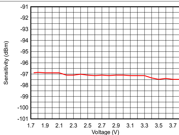
図 7-18. 感度と電源電圧 (VDDDS) との関係 (LE 1M PHY、2.44GHz)
