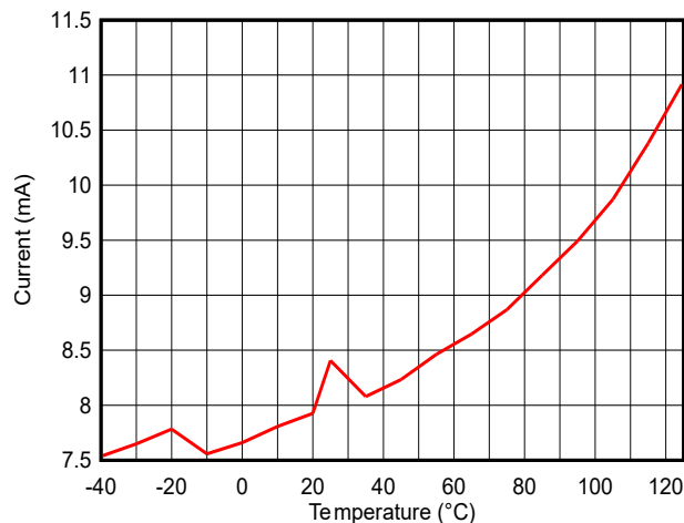
図 7-10. TX 電流と温度との関係 (LE 1M PHY、2.44GHz、0dBm)、VDD5 = 3.3V
