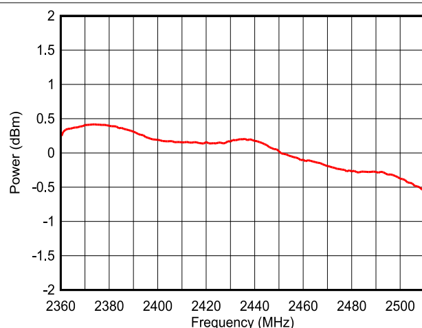
図 7-26. 出力電力と周波数との関係 (LE 1M PHY、0dBm)
