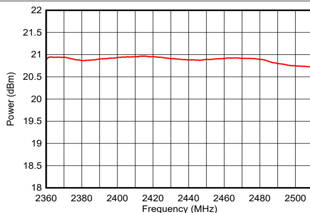
図 7-27. 出力電力と周波数との関係 (LE 1M PHY、+20dBm)
