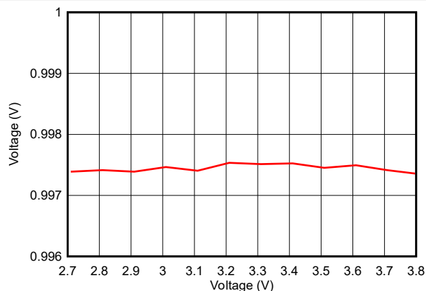
図 7-35. ADC 精度と電源電圧との関係 ( V_{in} = 1V、内部リファレンス、200ksps)
