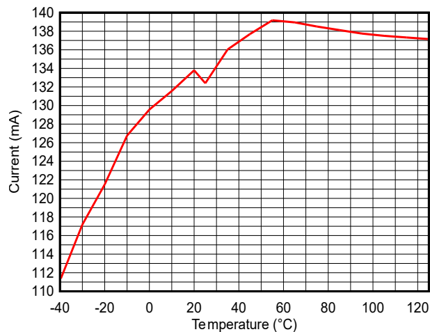
図 7-11. TX 電流と温度との関係 (LE 1M PHY、2.44GHz、20dBm)、VDD5 = 3.3V
