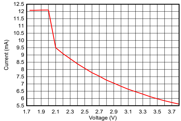
図 7-9. RX 電流と電源電圧 ( V_{DD5} ) との関係 (LE 1M PHY、2.44GHz)
