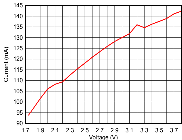
図 7-13. TX 電流と電源電圧 (VDD5) との関係 (LE 1M PHY、2.44GHz、+20dBm)
