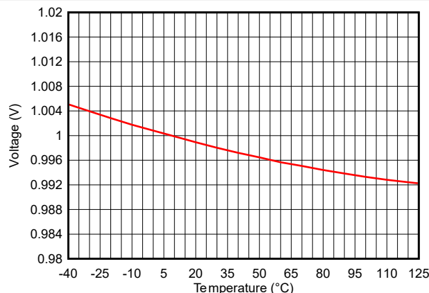
図 7-34. ADC の精度と温度との関係 ( V_{in} = 1V、内部リファレンス、200ksps)
