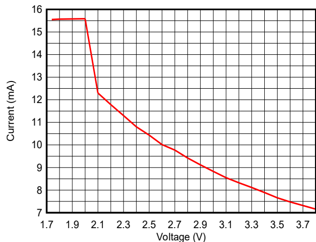
図 7-12. TX 電流と電源電圧 (VDD5) との関係 (LE 1M PHY、2.44GHz、0dBm)
