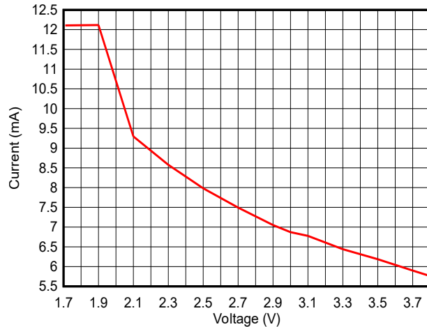
図 7-6. アクティブモード (マイコン) 電流と電源電圧 ( V_{DD5} ) との関係 (Core Mark 実行)
