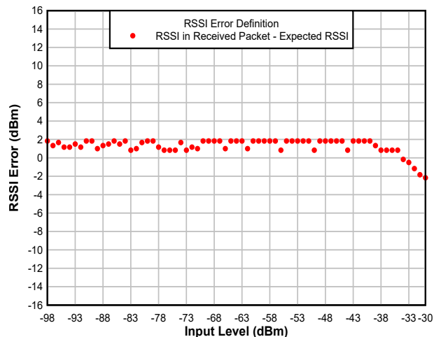
図 7-21. RSSI エラーと入力レベルとの関係 (dBm)
