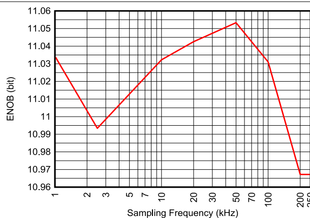
図 7-29. ENOB とサンプリング周波数との関係 ( V_{in} = 3V ランプ波、内部リファレンス、 F_{in} = F_s/10 )
