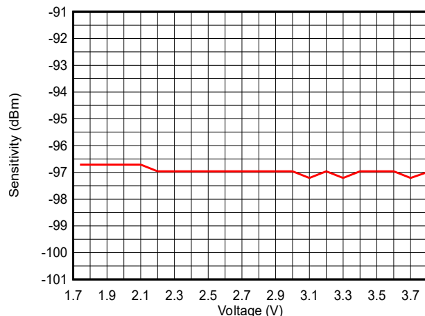
図 7-20. 感度と電源電圧 (VDD5) との関係 (LE 1M PHY、2.44GHz、DC/DC 無効)
