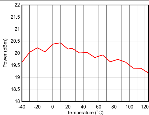
図 7-23. 出力電力と温度との関係 (LE 1M PHY、2.44GHz、20dBm)
