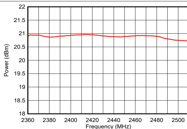
図 7-27. 出力電力と周波数との関係 (LE 1M PHY、+20dBm)
