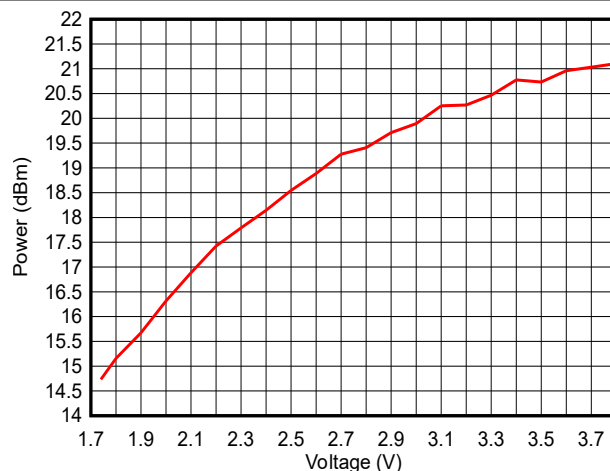
図 7-25. 出力電力と電源電圧 (VDDS) との関係 (LE 1M PHY、2.44GHz、+20dBm)
