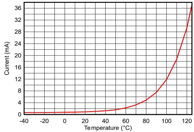
図 7-7. スタンバイモード (マイコン) の電流と温度との関係 (SRAM および部分的レジスタ保持、RTC イネーブル、 V_{DD5} = 3.3\text{V} )
