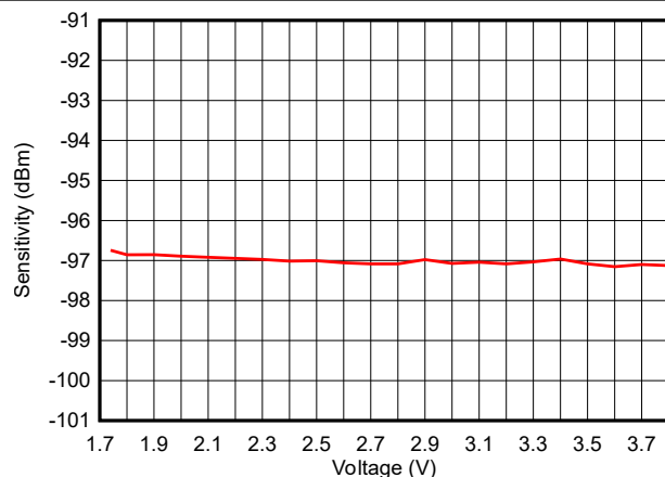
図 7-18. 感度と電源電圧との関係 (VDDSD) (BLE 1Mbps, 2.44GHz)
