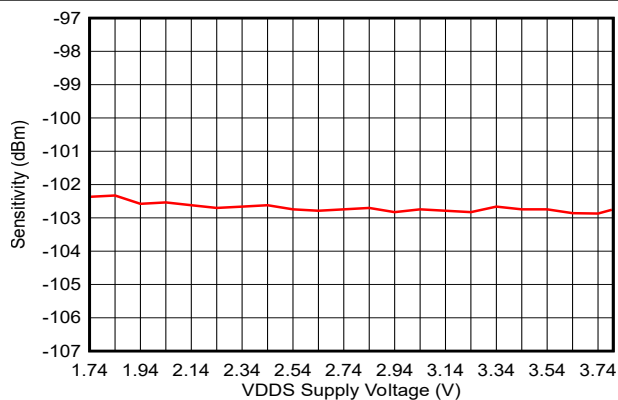
図 7-19. 感度と VDDSD との関係 (IEEE 802.15.4 PHY)
