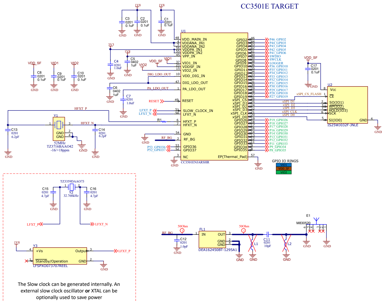
図 8-1. CC350xE のリファレンス回路図
