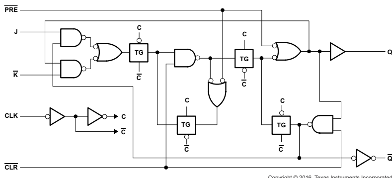
ロジック図
