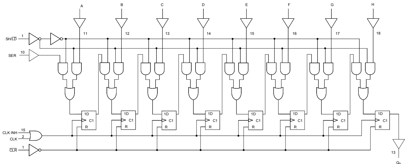
機能ダイアグラム
