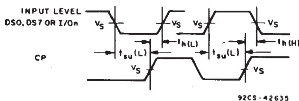
図 5-4. データの前提条件時間
