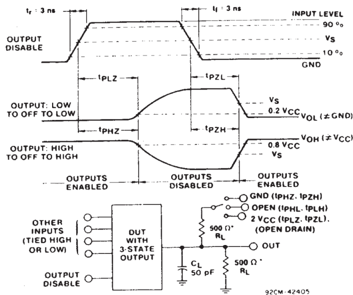
図 5-3. 3 ステート伝搬遅延時間とテスト回路
