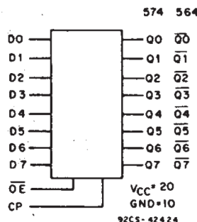
機能ブロック図
