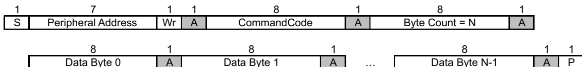
図 7-5. ブロック書き込みプロトコル
