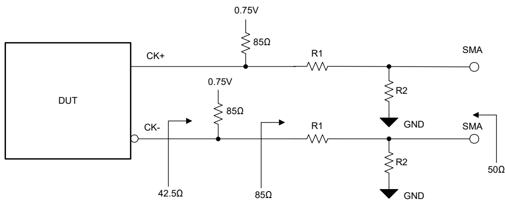
図 6-1. AC テスト負荷 (Intel DB2000QL ドキュメント参照)
