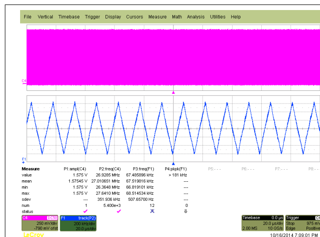
図 9-6. f_{OUT} = 27\text{MHz} 、VCO 周波数 < 125MHz、SSC (センター 2%)
