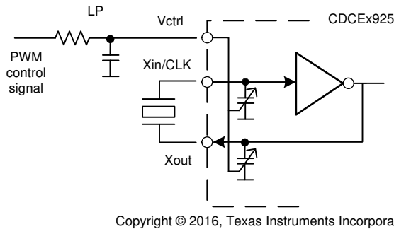
図 9-5. PWM 入力を使用した VCXO 制御の周波数調整
