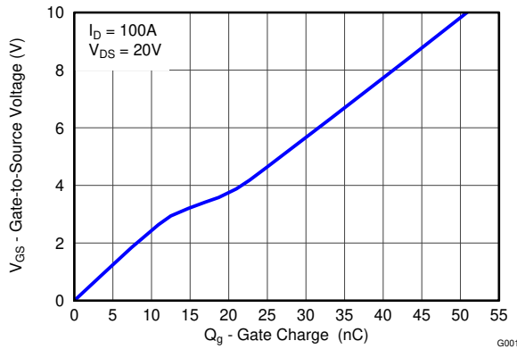
図 4-4. Gate Charge
