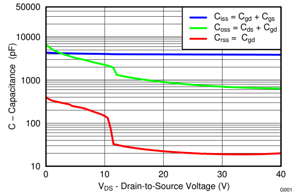
図 4-5. Capacitance
