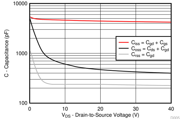
図 4-5. Capacitance
