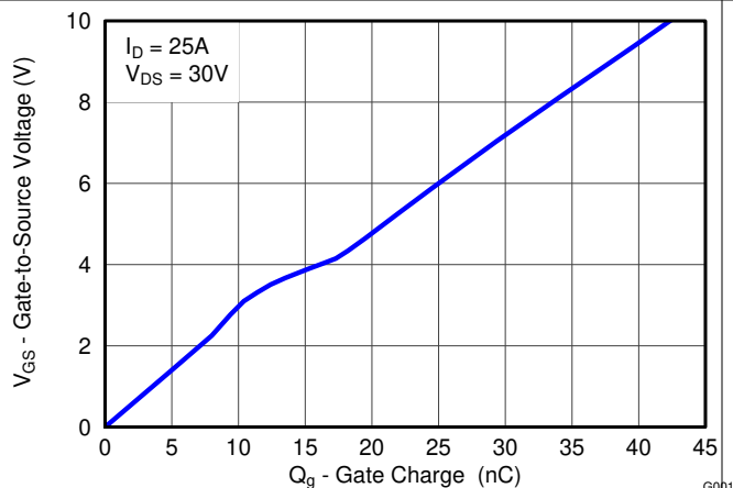
図 4-4. ゲート電荷
