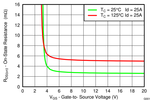
R_{DS(on)} と V_{GS} との関係
