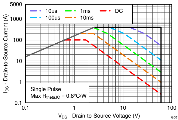
図 4-10. 安全動作領域 (最大値)
