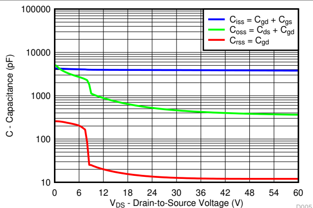
図 4-5. 容量
