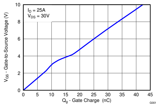
ゲート電荷
