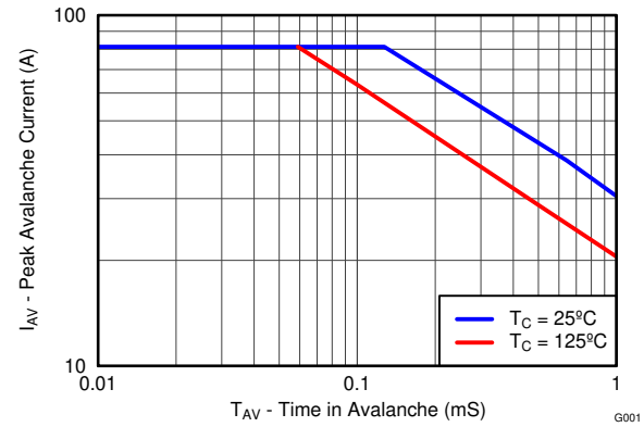
図 4-11. 単一パルスの非クランプ誘導性スイッチング
