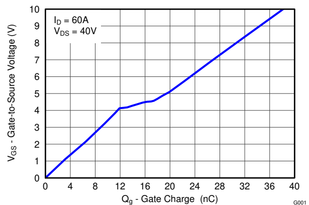
ゲート電荷
