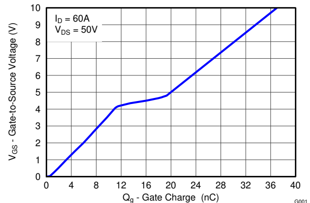
ゲート電荷
