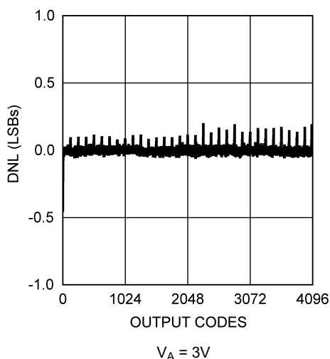
图 5-2. DNL vs Output Code
