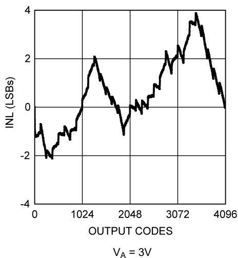
图 5-4. INL vs Output Code
