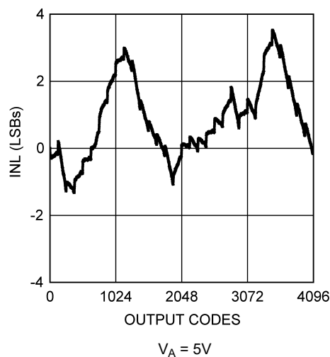
图 5-5. INL vs Output Code
