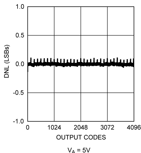
图 5-3. DNL vs Output Code
