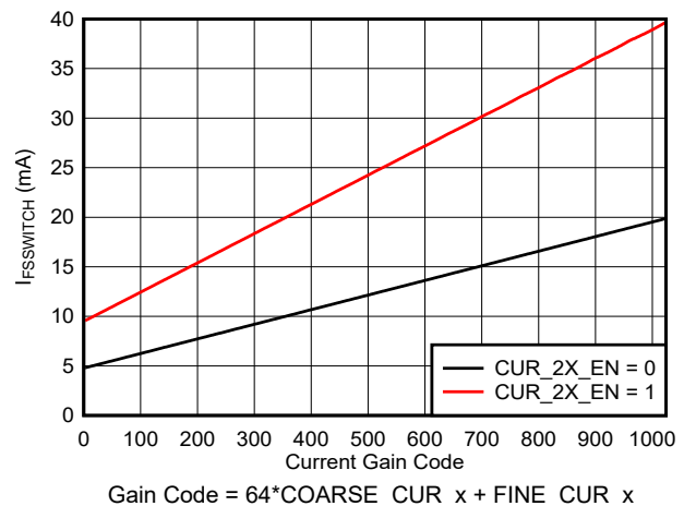
图 6-15. I_{\text{FS\_SWITCH}} vs Gain Code
