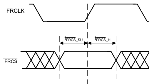
図 6-7. \overline{\text{FRCS}} Timing Diagram
