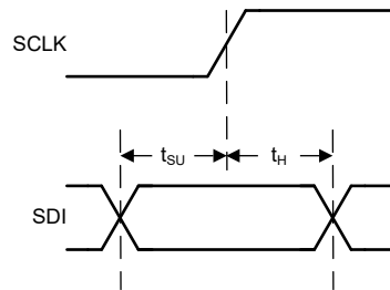
図 6-2. SPI Data Input Timing Diagram
