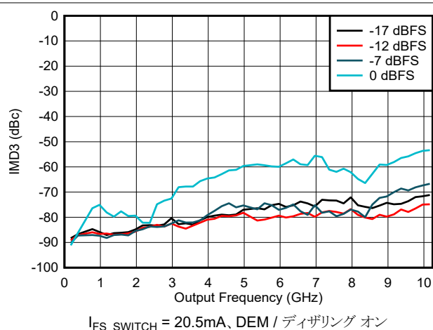
図 6-133. NRZ/RF モードにおける IMD3 と周波数およびデジタル振幅との関係
