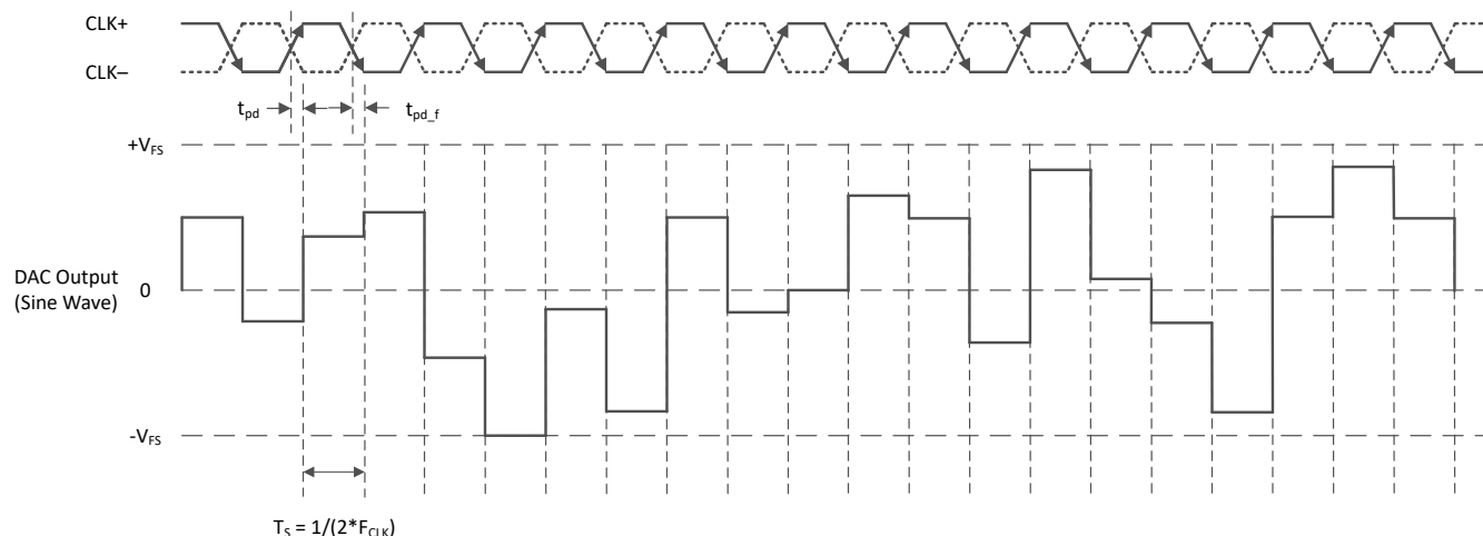
図 7-9. DES モードのタイミング図
