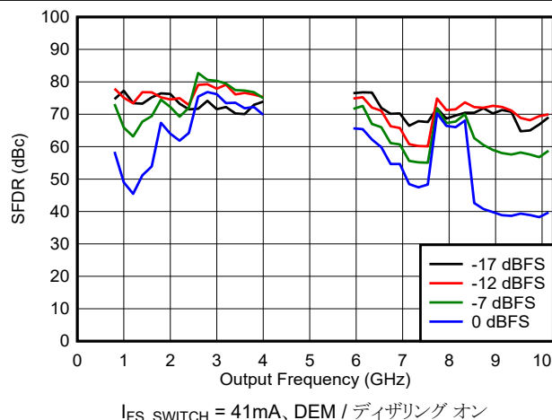
図 6-123. DES2X モードでの SFDR と周波数およびデジタル振幅との関係
