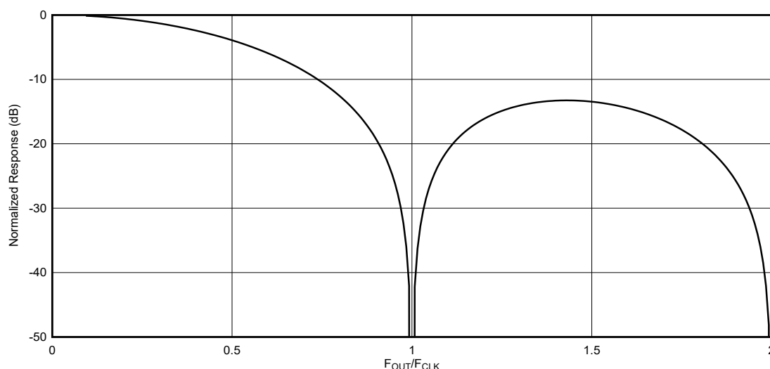
図 7-4. NRZ モード出力周波数応答
