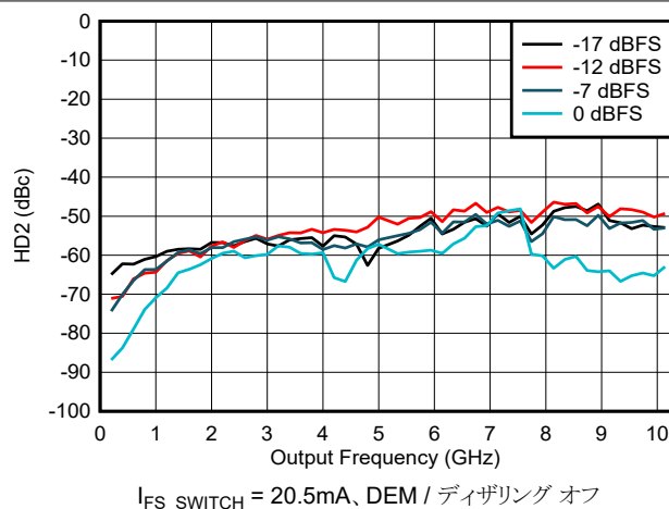
図 6-160. NRZ/RF モードにおける HD2 と周波数およびデジタル振幅との関係
