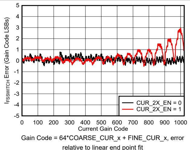
図 6-17. I_{\text{FS\_SWITCH}} Error vs Gain Code
