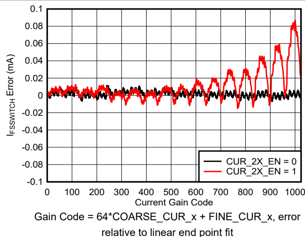
図 6-16. I_{\text{FS\_SWITCH}} Error vs Gain Code
