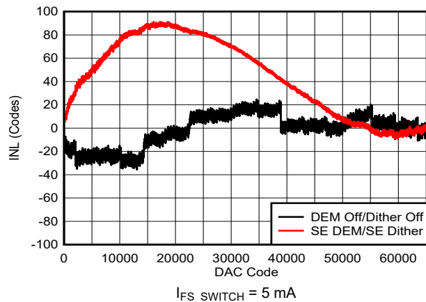
図 6-14. INL vs DAC Code: 5 mA
