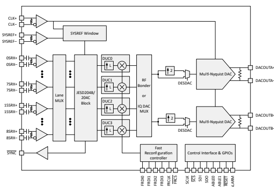
ブロック図
