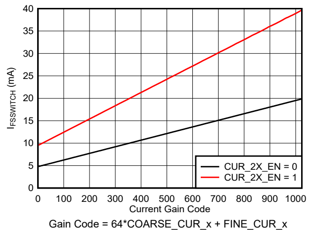
図 6-15. I_{\text{FS\_SWITCH}} vs Gain Code
