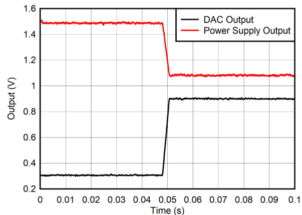
图 9-6. Power Supply Margin Low
