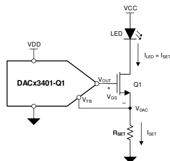
DACx3401-Q1 による LED バイアス印加
