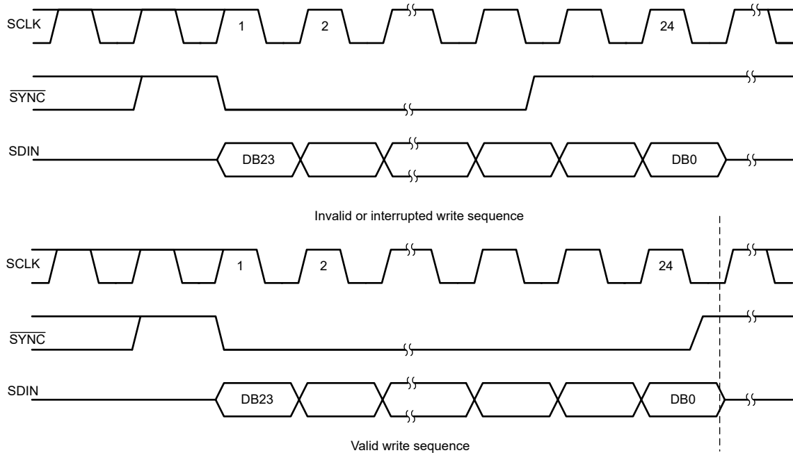
图 7-3. \overline{\text{SYNC}} Interrupt
