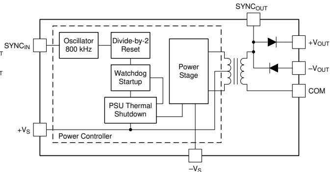
デュアル出力のブロック図
