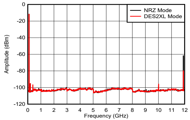
図 6-9. f_{\text{OUT}} = 97\text{MHz} , -6dBFS
