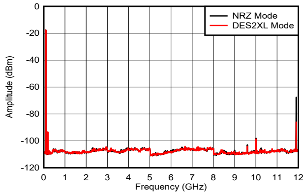
図 6-8. f_{\text{OUT}} = 97\text{MHz} , 0dBFS
