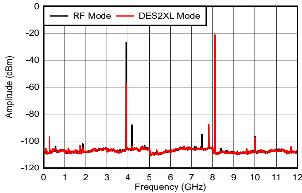
図 6-20. f_{\text{OUT}} = 8097\text{MHz} , 0dBFS
