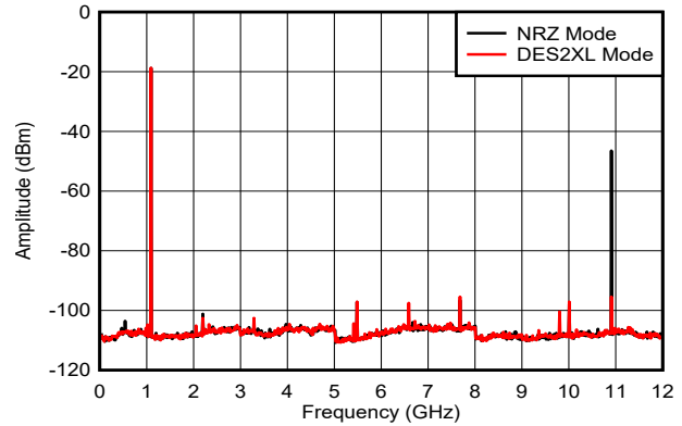
図 6-11. f_{\text{OUT}} = 1097\text{MHz} , 0dBFS
