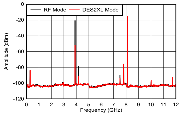
図 6-21. f_{\text{OUT}} = 8097\text{MHz} , -6dBFS
