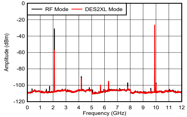
図 6-23. f_{\text{OUT}} = 9897\text{MHz} , 0dBFS
