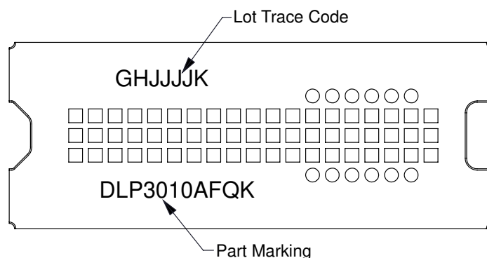
図 11-2. DMD Marking
