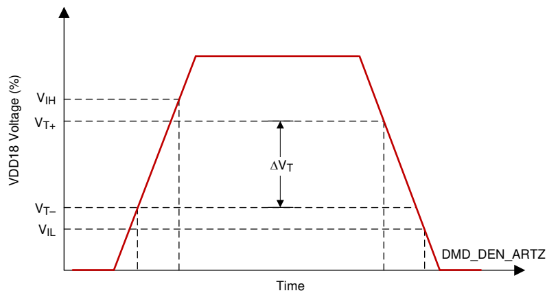
図 5-8. LVCMOS Input Hysteresis
