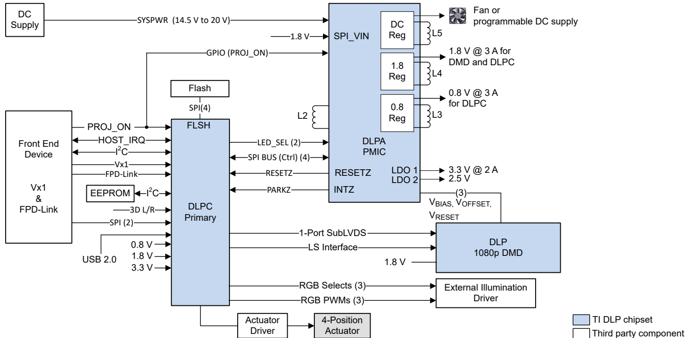
図 7-1. 外部照明ドライバを使用した代表的な 1080p システム図
