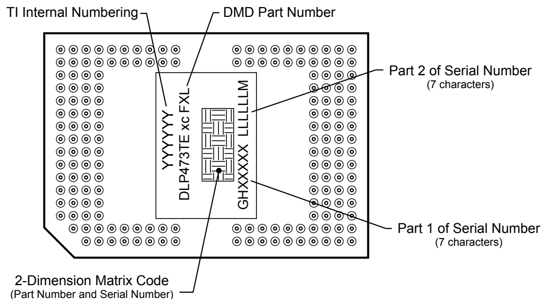
図 9-2. DMD のマーキング位置
