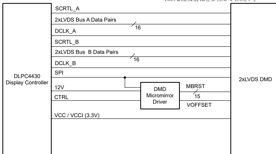
DLP650LE のアプリケーション概略図
