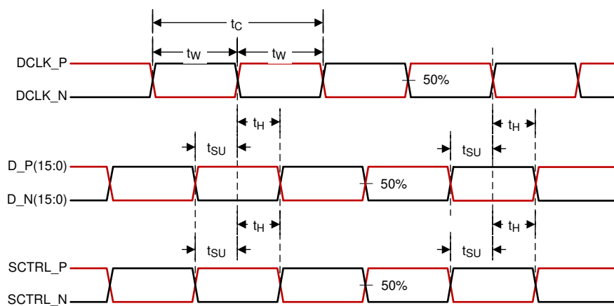
図 6-6. Timing Requirements
