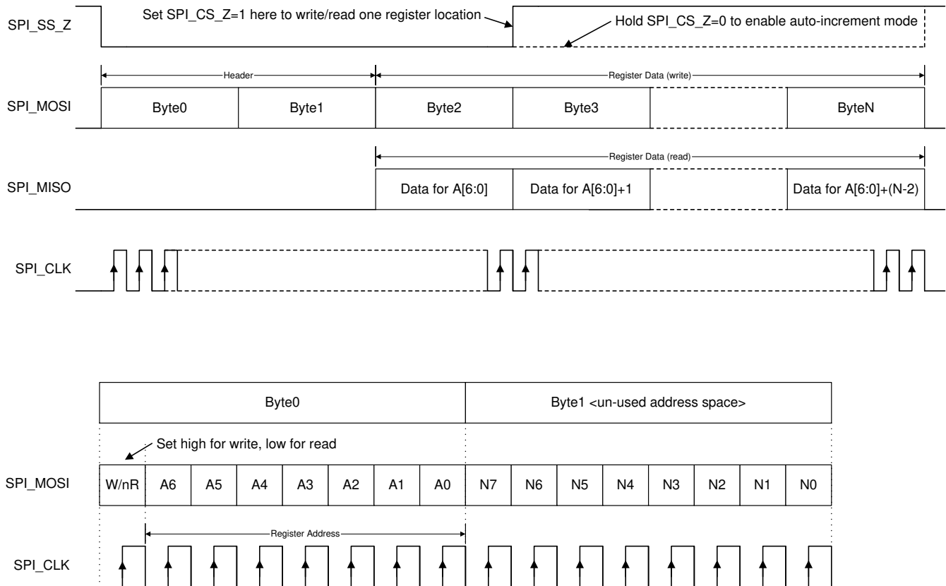
図 6-10. SPI Protocol
