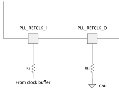
図 8-1. クロック発振器に必要なディスクリート部品
