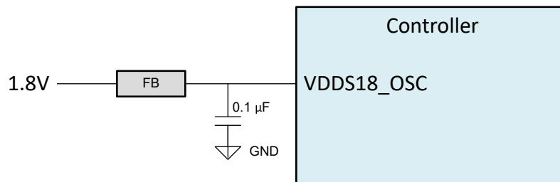
図 8-2. クロック発振器の電源フィルタリング
