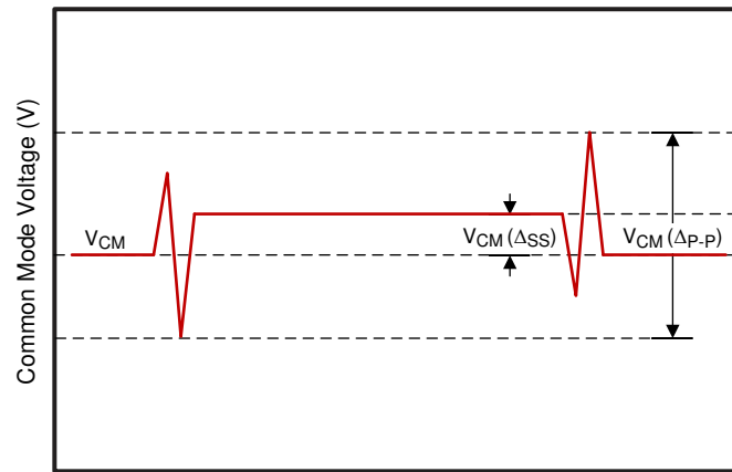
図 5-2. 同相電圧
