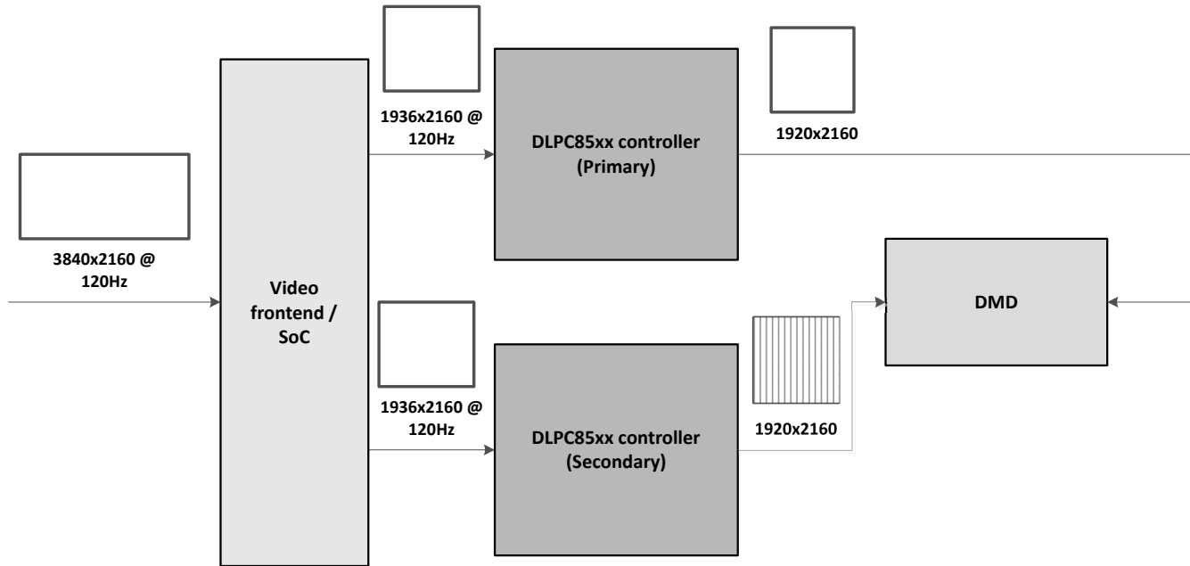
図 6-2. ビデオ入力解像度を含めたシステム ブロック図
