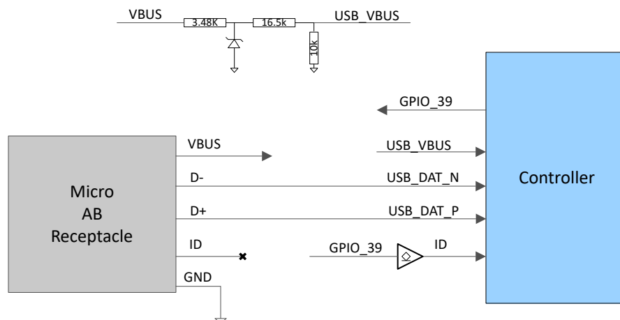
図 5-5. DLPC8545 コントローラの USB の使用例
