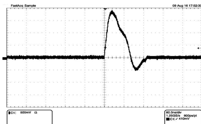
6-10. 10Base-T Link Pulse
