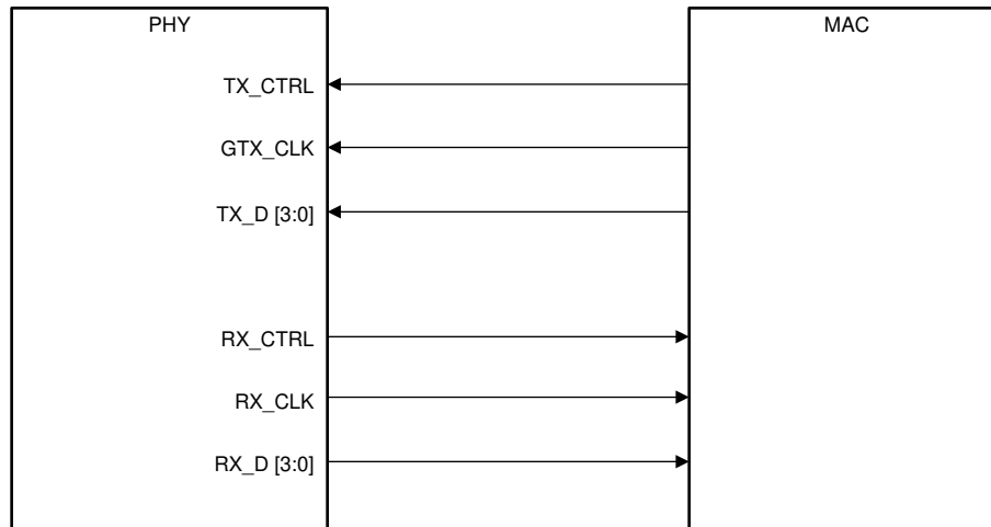
图 7-4. RGMII Connections
