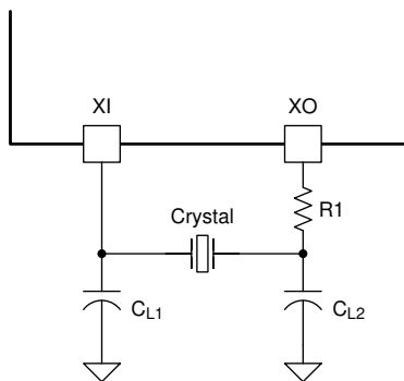
図 9-4. 水晶発振回路
