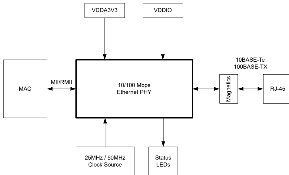
図 9-1. DP83826Ax の代表的なアプリケーション
