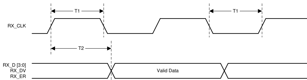
図 7-7. 100m MII 受信タイミング
