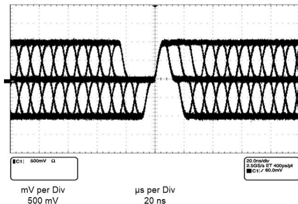
図 7-13. 100BASE-TX PMD アイ波形
