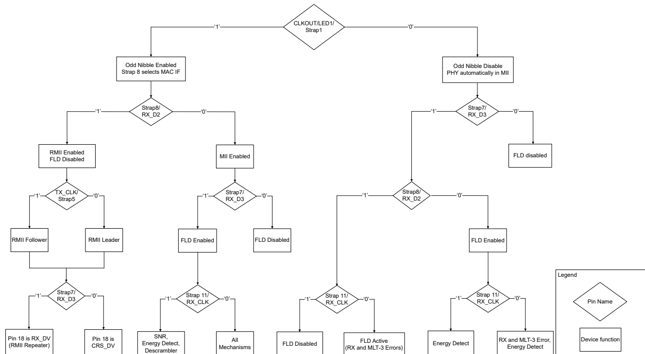
図 8-13. 拡張ブートストラップフローチャート
