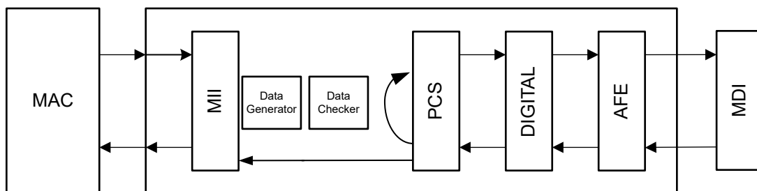
図 7-10. データ ジェネレータなしのリバース ループバック
