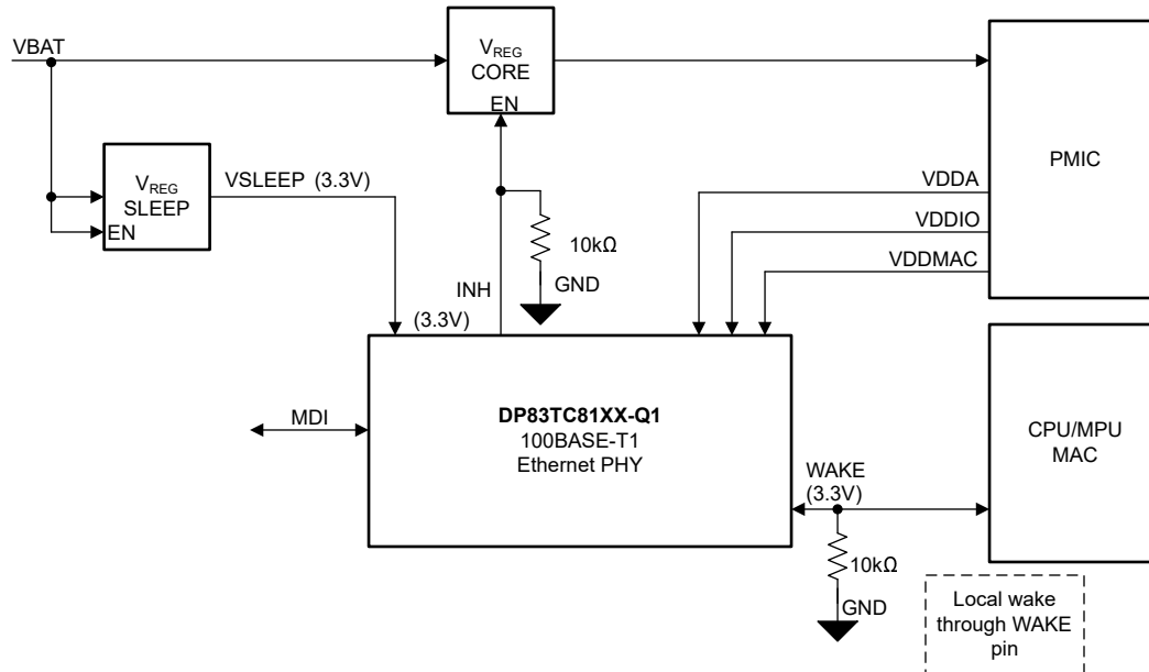
図 7-13. TC10 システム例 — ローカル ウェイク
