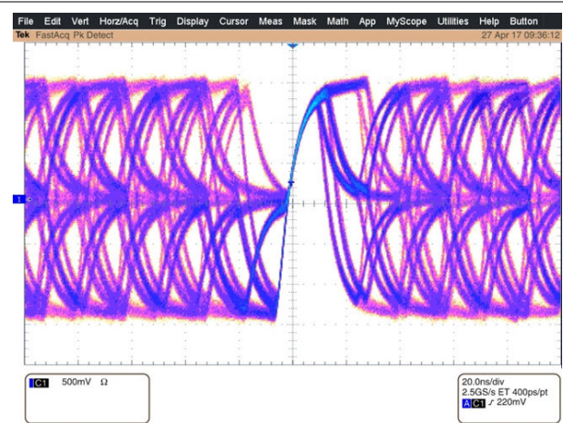
図 9-8. MDI アイドル ストリーム (可変永続性)
