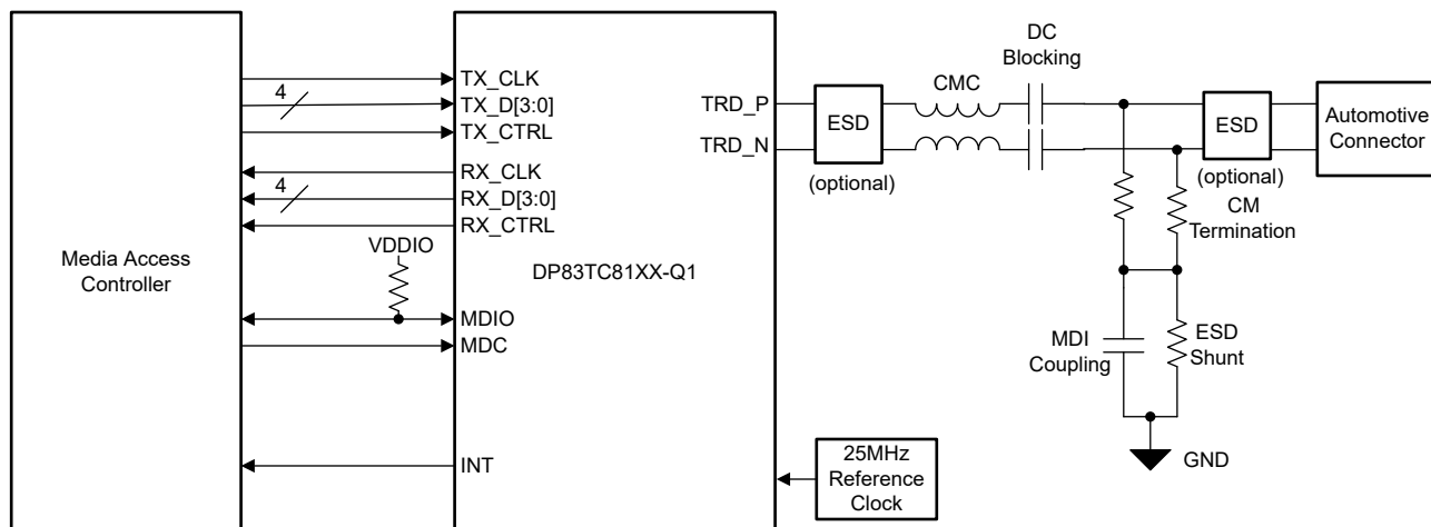
図 9-5. 代表的なアプリケーション (RGMII)
