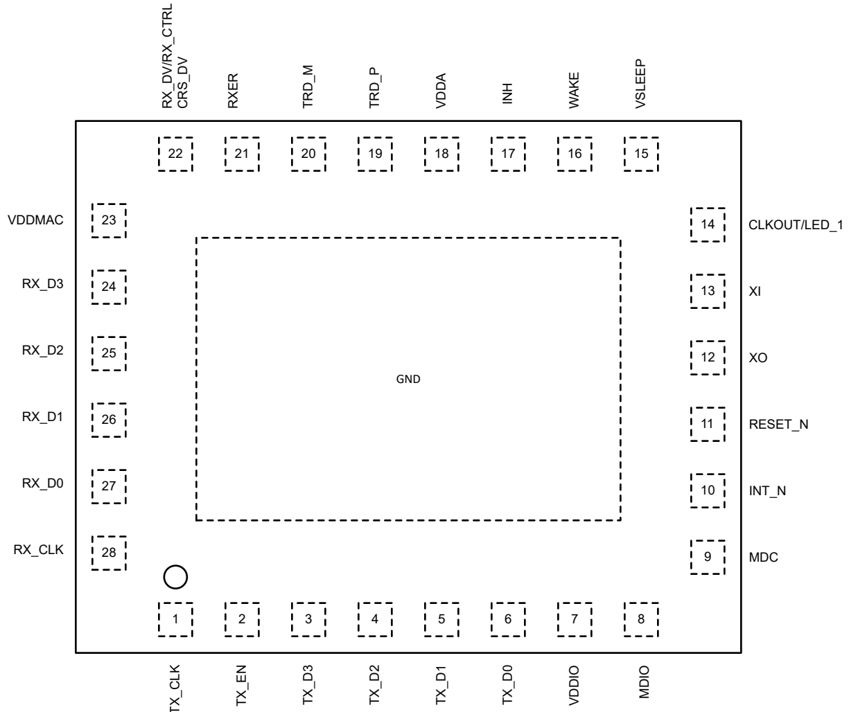
図 5-2. DP83TC813R-Q1 RHF パッケージ 28-ピン VQFN 上面図
