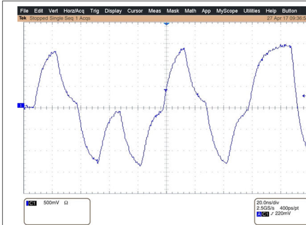
図 9-7. MDI アイドル ストリーム
