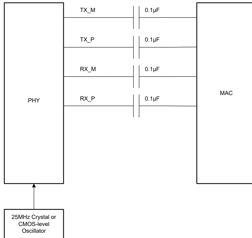
図 7-14. SGMII の接続
