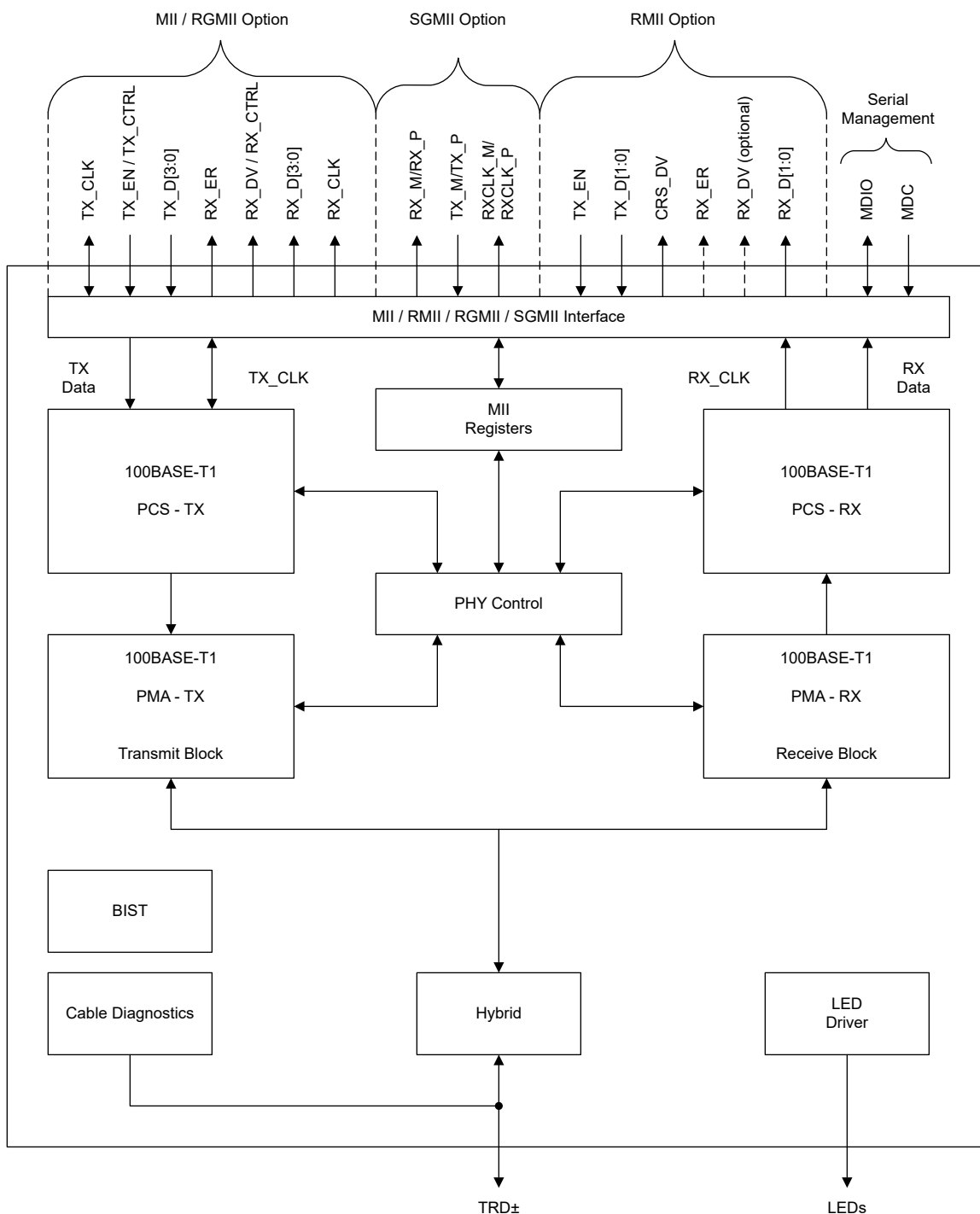
図 7-1. DP83TC814S-Q1
