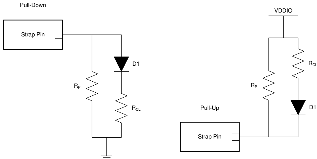
図 7-17. ストラップ接続の例
