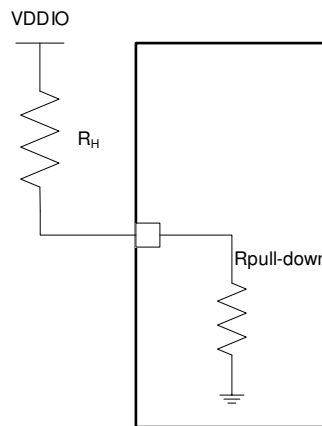
図 7-16. ストラップ回路
