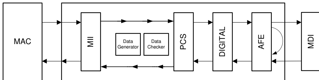
図 7-2. すべてのループバック
