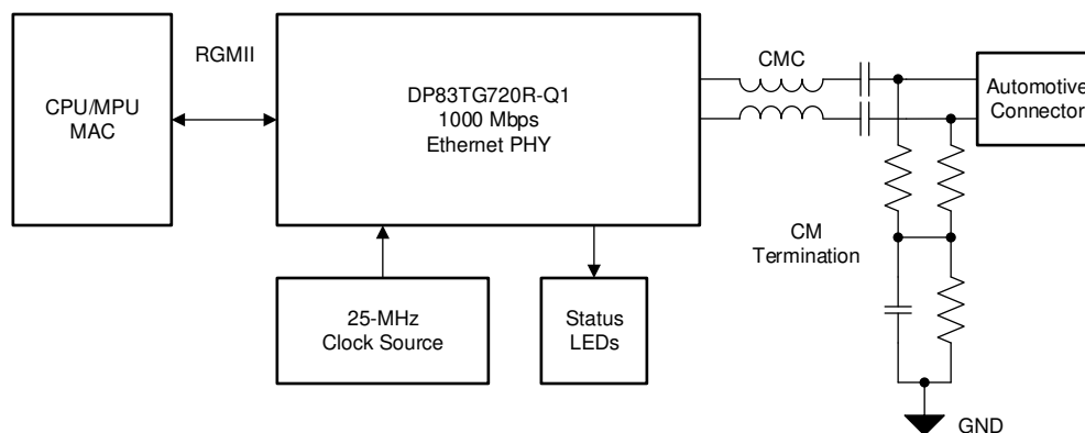
概略回路図
