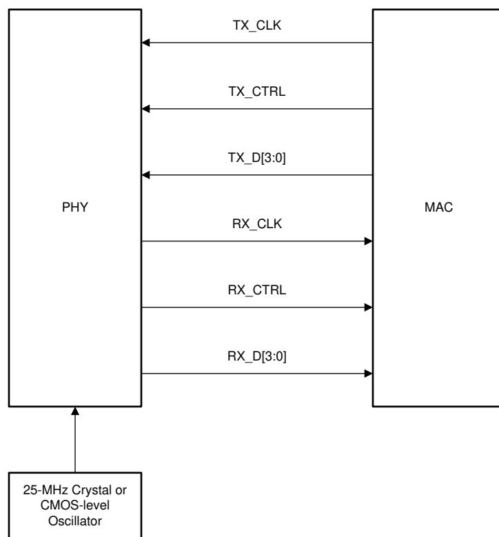
図 7-13. RGMII の接続
