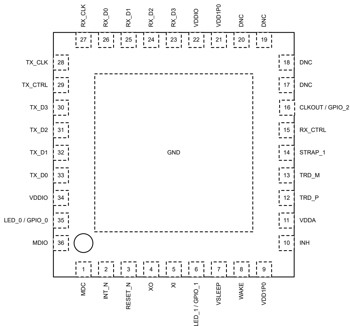
図 5-1. RHA パッケージ 36 ピン VQFN 上面図
