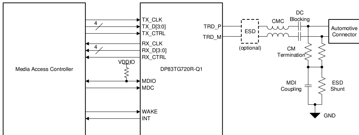
図 8-1. 代表的なアプリケーション (RGMII)
