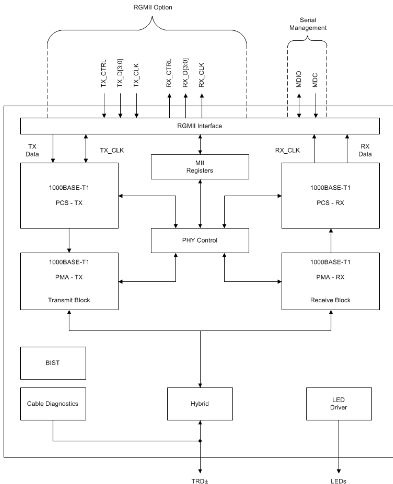
図 7-1. DP83TG720R-Q1 の機能ブロック図
