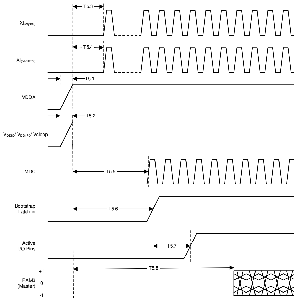
図 6-1. 起動タイミング
