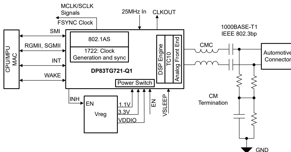
概略回路図
