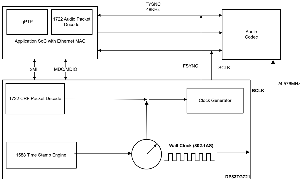
図 5-3. DP83TG721-Q1 を使用したオーディオ オーバー イーサネット アーキテクチャ
