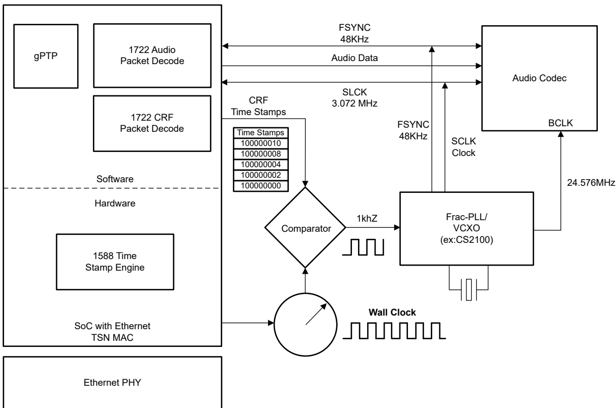
図 5-2. 代表的なオーディオ オーバー イーサネット アーキテクチャ
