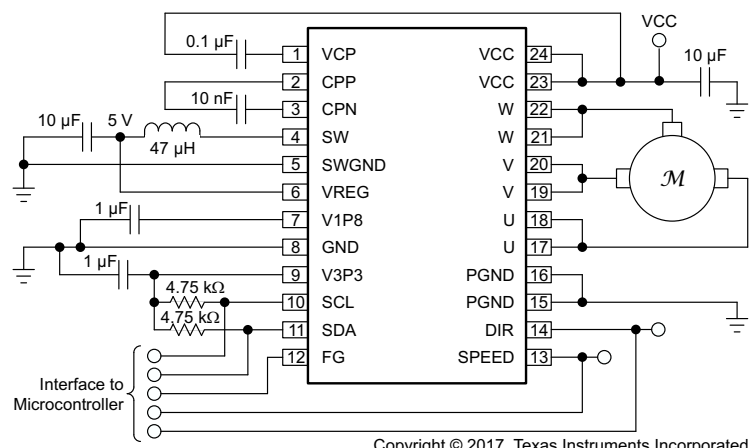
アプリケーション回路図
