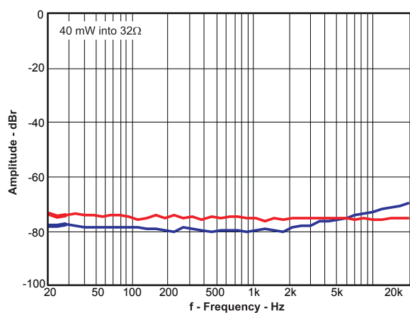
図9. チャネル・セパレーション
