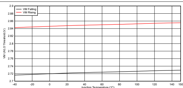
図 6-7. VM UVLO スレッシュホールド
