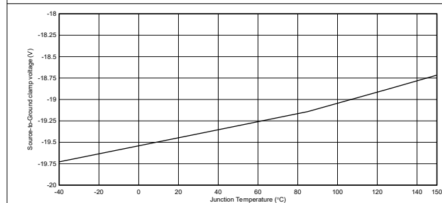
図 6-6. ソース-グランド間クランプ電圧
