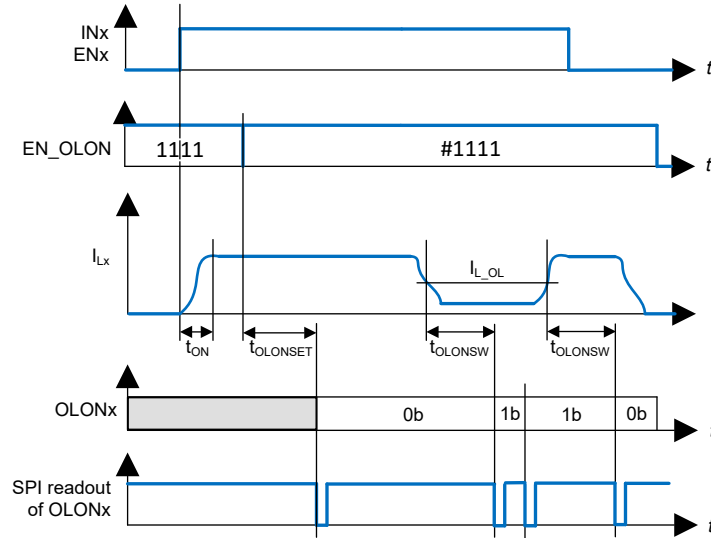
図 7-17. オン時の開放負荷 (直接チャンネル診断)
