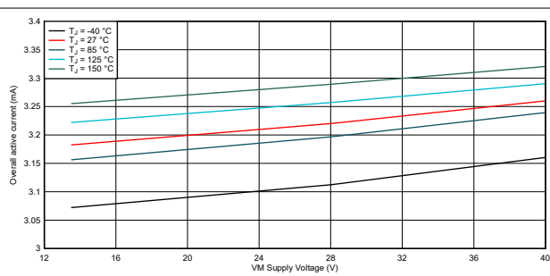
図 6-3. アクティブモードの電源電流、VDD = 5.5V
