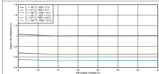
図 6-4. スイッチ オン抵抗
