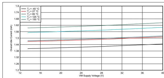
図 6-2. アイドルモード消費電流、VDD = 5.5V
