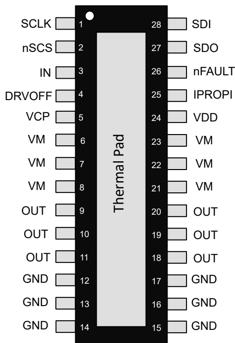
図 5-3. DRV8143P-Q1 SPI (P) バリエーション、HVSSOP (28) パッケージ
