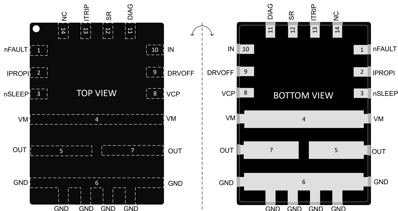
図 5-1. DRV8143H-Q1 HW バリエーション、VQFN-HR (14) パッケージ
