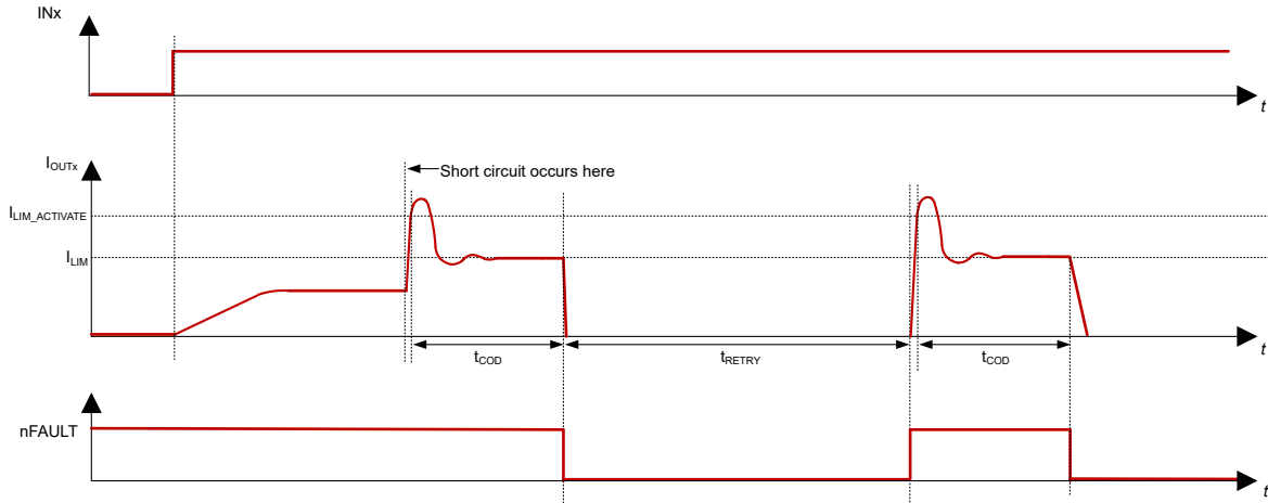
図 6-10. COD イネーブルの場合の短絡に対する電流制限回路の応答
