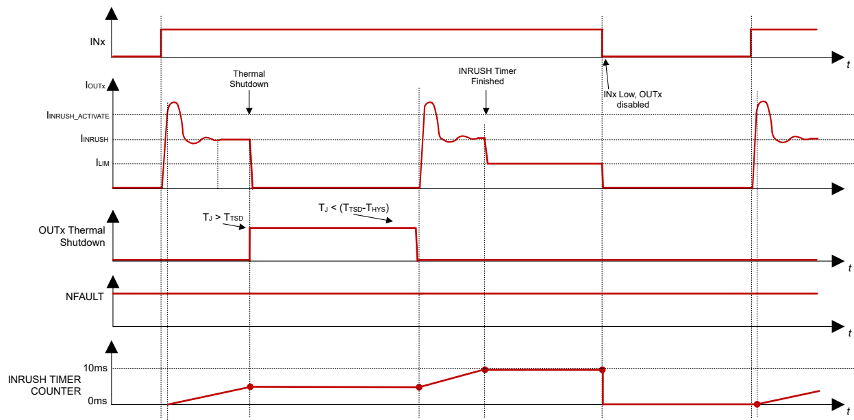
図 6-12. t_{INRUSH} 中のチャネル サーマル シャットダウンによる INRUSH タイマの例
