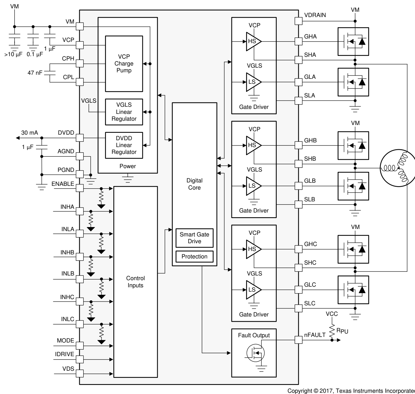
図 8-1. DRV8320H のブロック図
