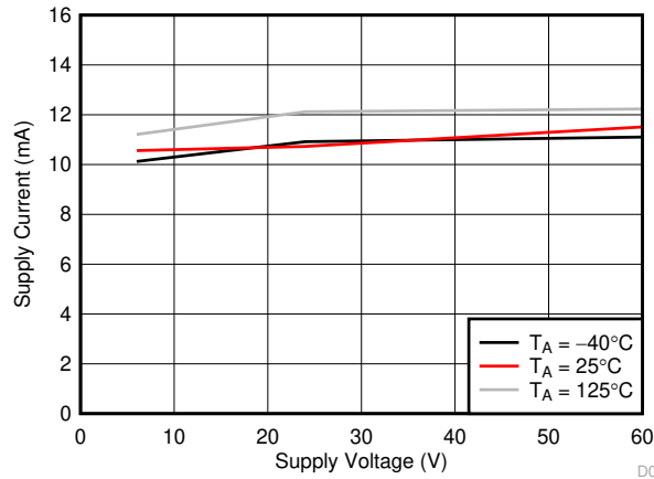
図 7-2. 電源電流と VM との関係
