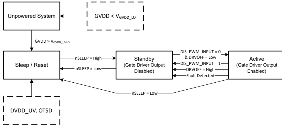
図 6-22. 機能状態図
