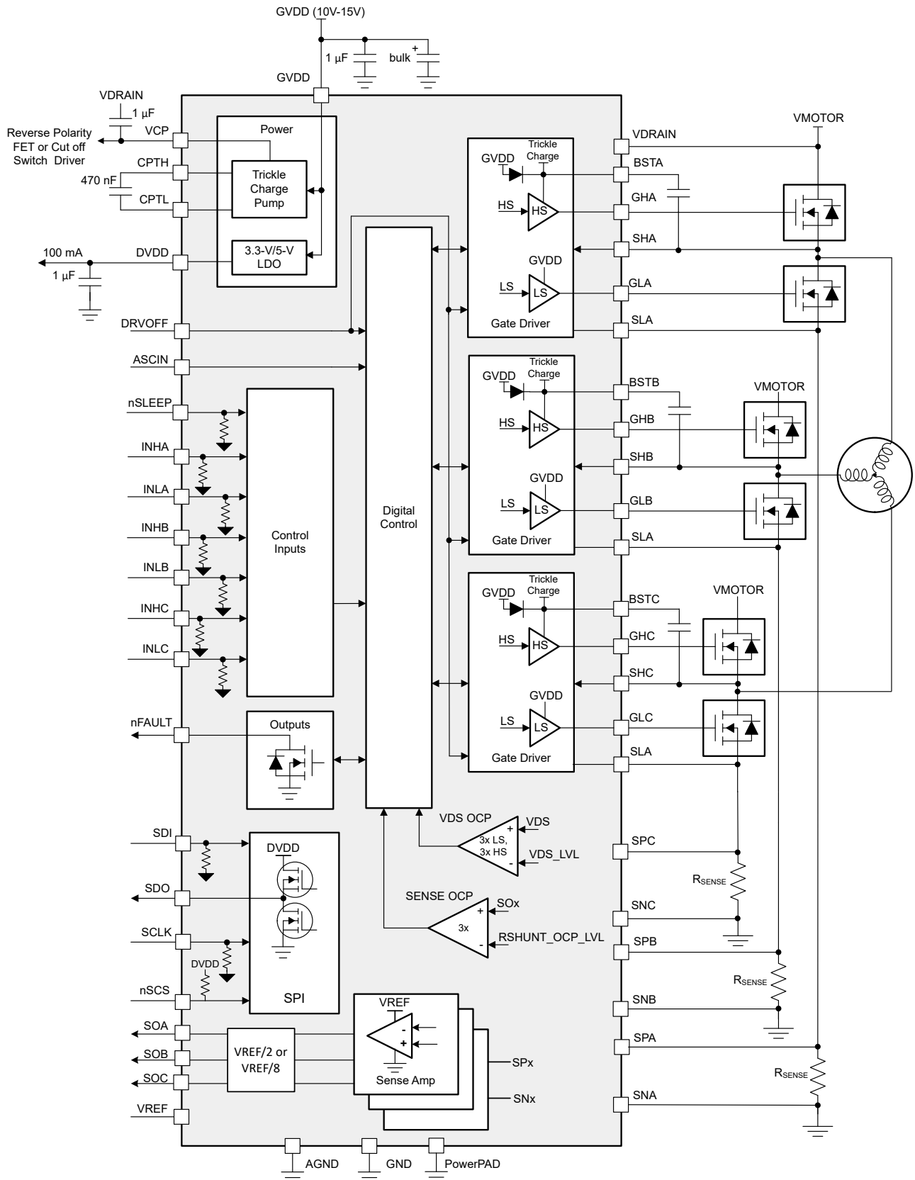
図 6-1. DRV8363-Q1 のブロック図
