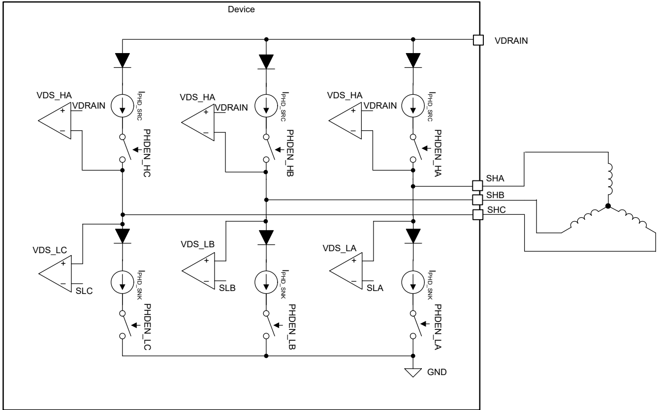
図 6-21. 位相診断
