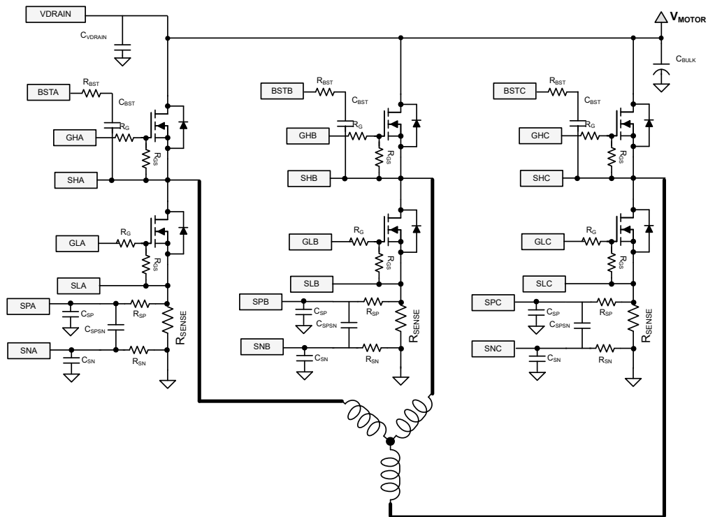
図 7-1. DRV8363-Q1 の代表的なアプリケーション回路
