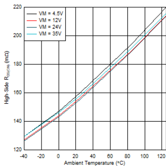
図 6-9. ハイスайд R_{DS(ON)} 温度特性
