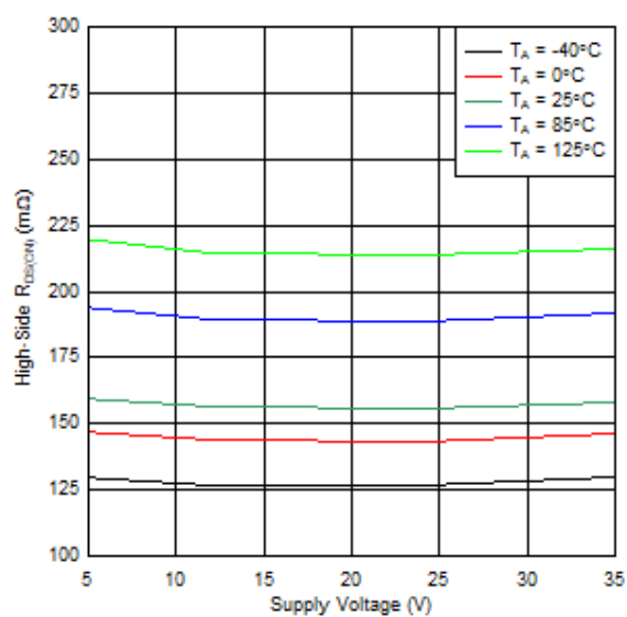
図 6-8. ハイスайд R_{DS(ON)} と電源電圧
